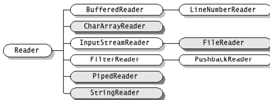
FIGURE 3 – Flux texte, c’est-à-dire de caractères, en entrée (source SUN).
