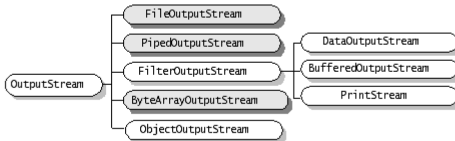
FIGURE 2 – Flux binaires, c’est-à-dire d’octets, en sortie (source SUN).
