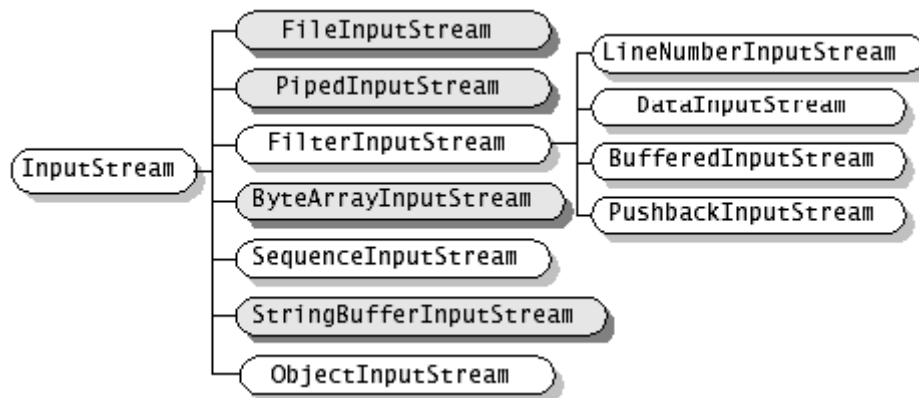
FIGURE 1 – Flux binaires, c’est-à-dire d’octets, en entrée (source SUN).
