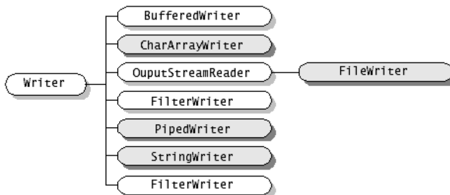
FIGURE 4 – Flux texte, c’est-à-dire de caractères, en sortie (source SUN). Attention : la troisième classe à partir du haut est OutputStreamWriter et non OutputStreamReader ; la classe PrintWriter pourrait également apparaître ici (sur fond blanc).
